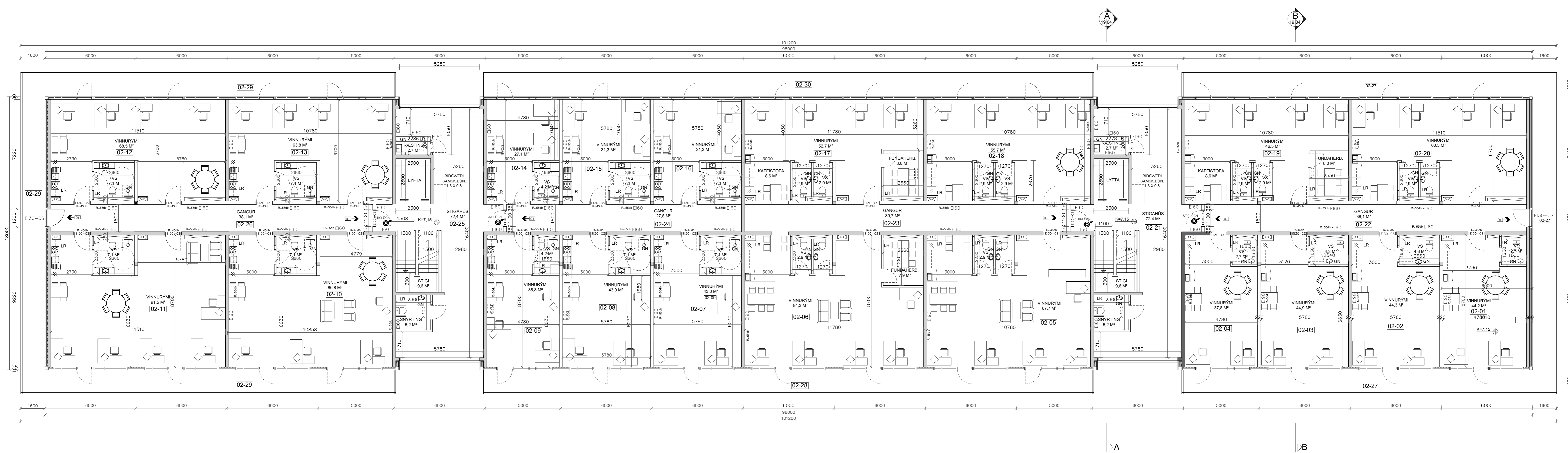
GRUNNMYND 2.HÆÐ MKV. 1:100
