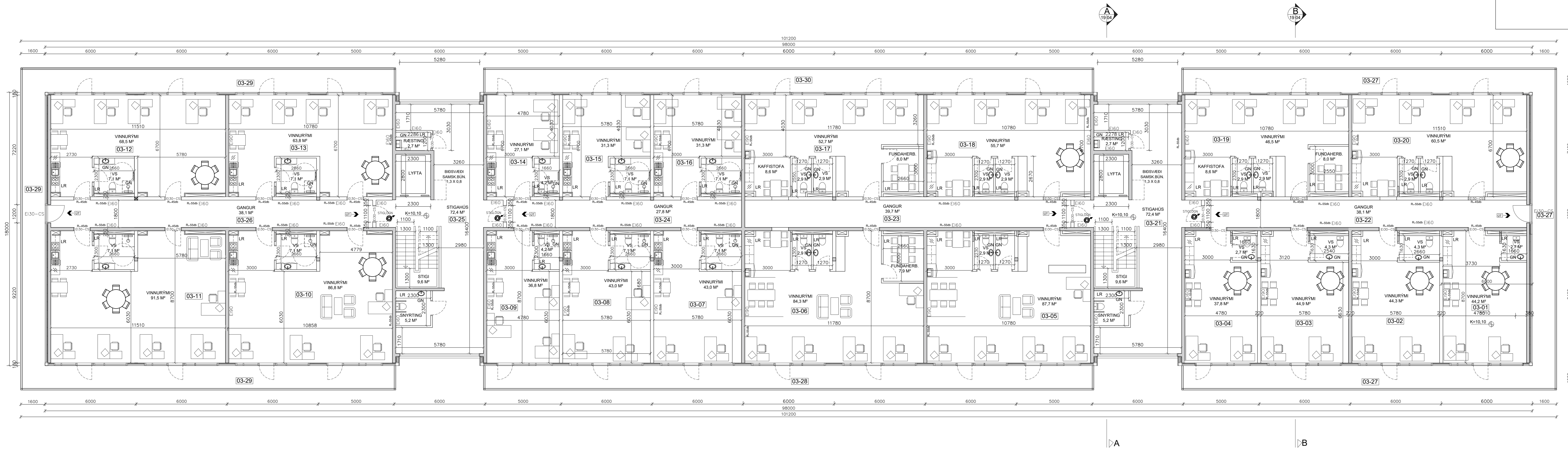
GRUNNMYND 3.HÆÐ MKV. 1:100
