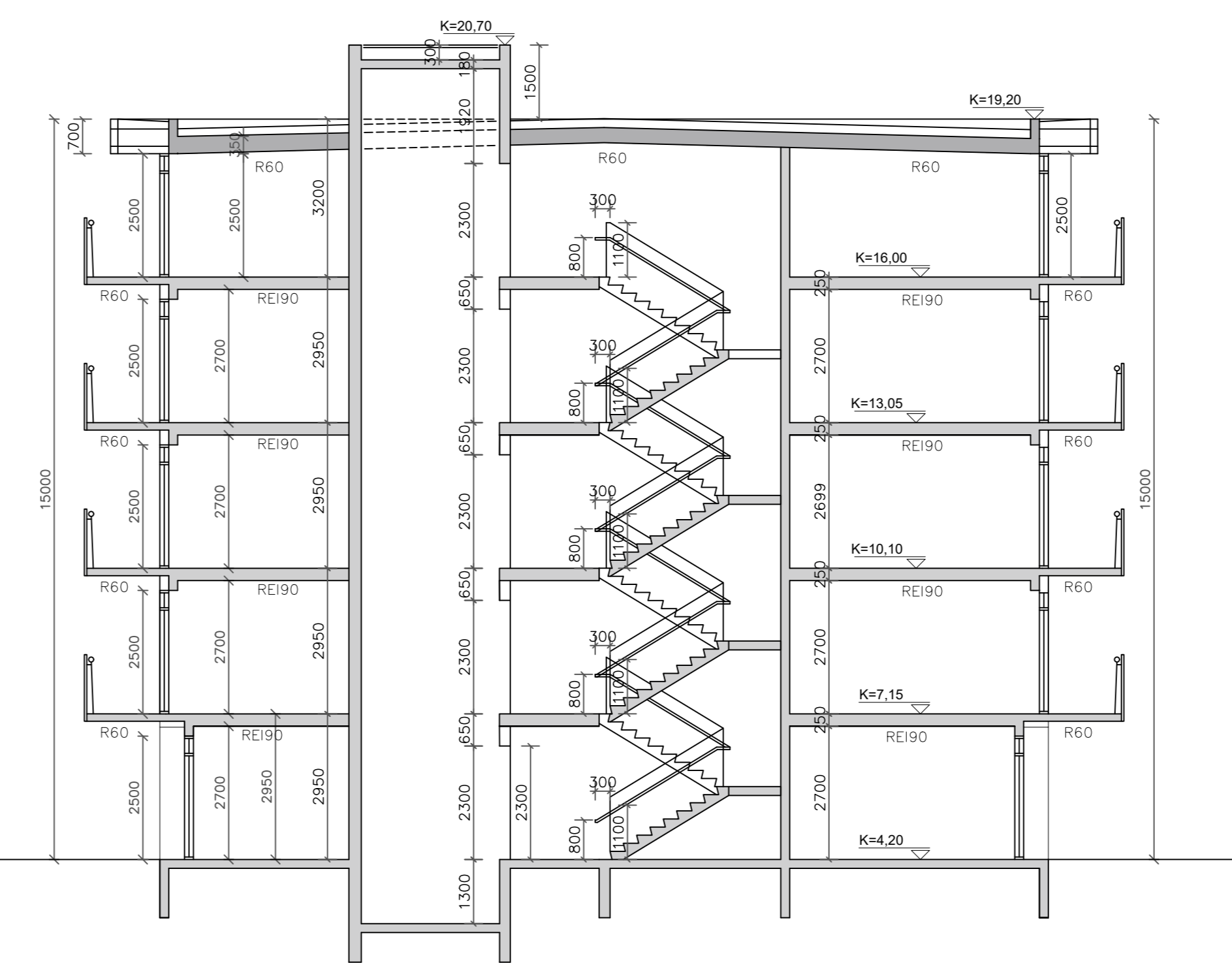
SNID A-A MKV. 1:100
